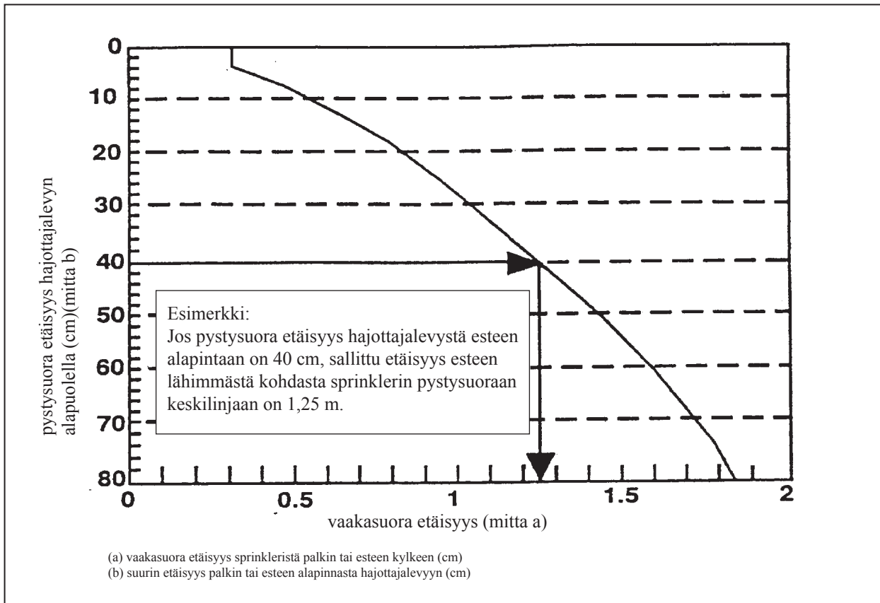
Kuva L5 – ESFR sprinklerien vaakasuora ja pystysuora etäisyys (cm) palkkiin tai esteeseen nähden
