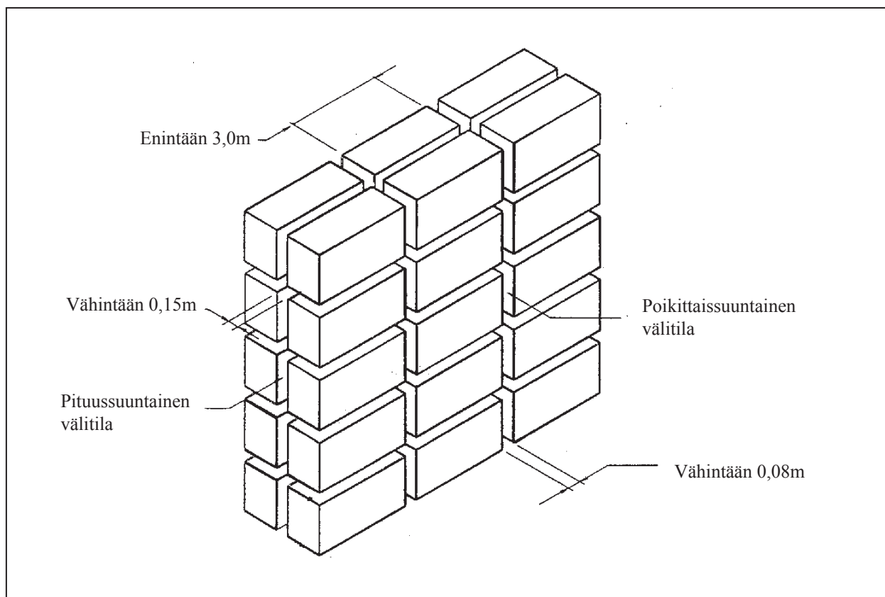
Kuva L1 - Varastointitapojen ST2, ST3 ja ST4 poikittaissuuntaiset ja pituussuuntaiset välitilat
